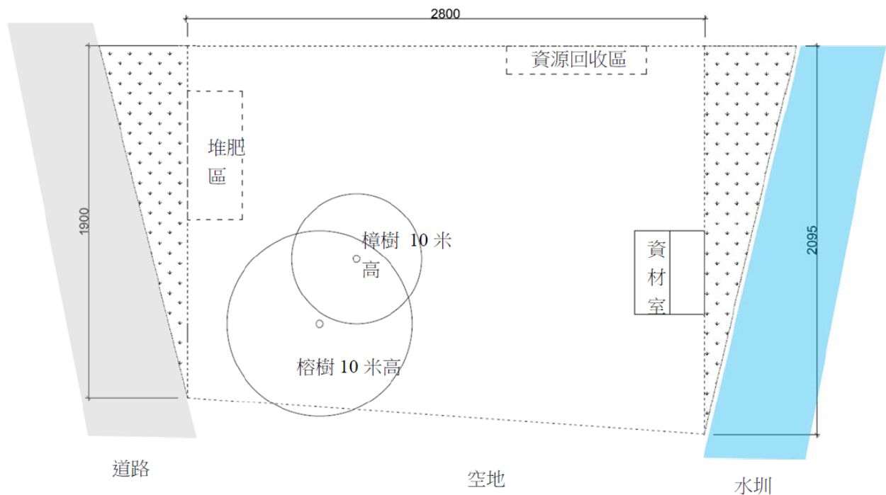
圖 基地現況與測量圖 (單位:公分)
