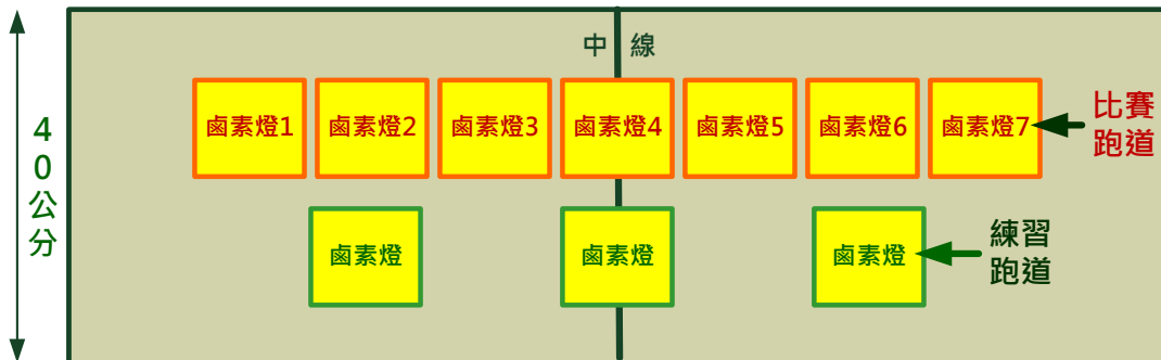
比賽跑道之鹵素燈功率為500W，距離比賽平面高度25公分，總共七個密集橫放
